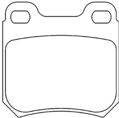
T1016
